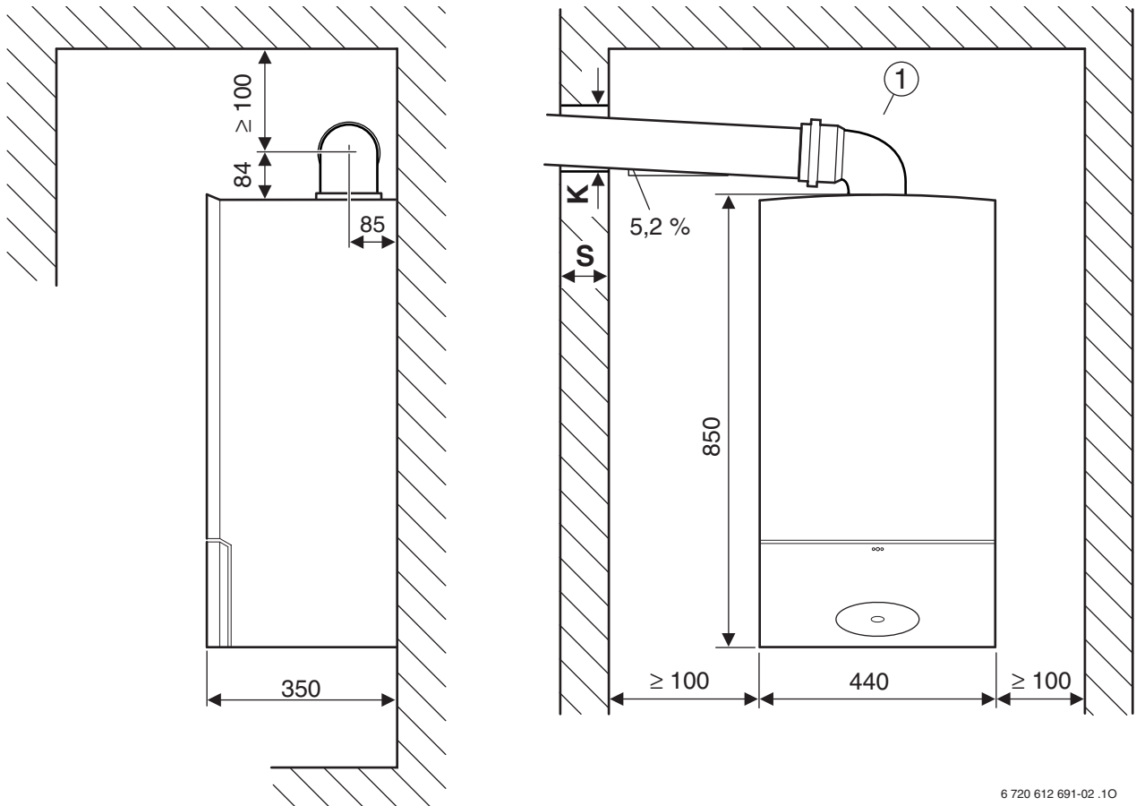
Fig. 6 Accessori Ø 60/100 mm
