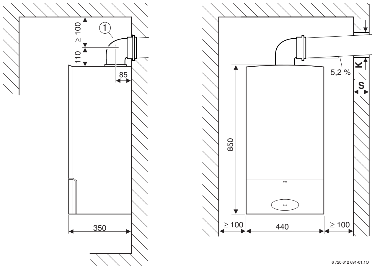
Fig. 5 Accessori Ø 80/125 mm oppure accessori Ø 80 mm
